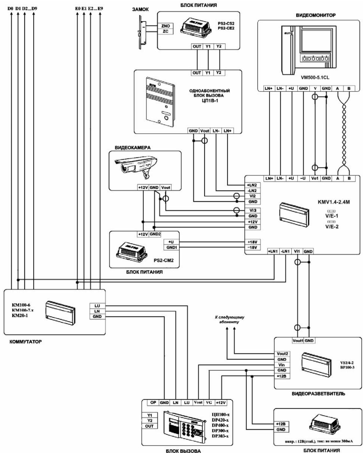
Рис.11. Пример схемы подключения видеомонитора к одноабонентному переговорному устройству и многоабонентному блоку вызова совместно с коммутатором КМВ1.4-2.4М.
