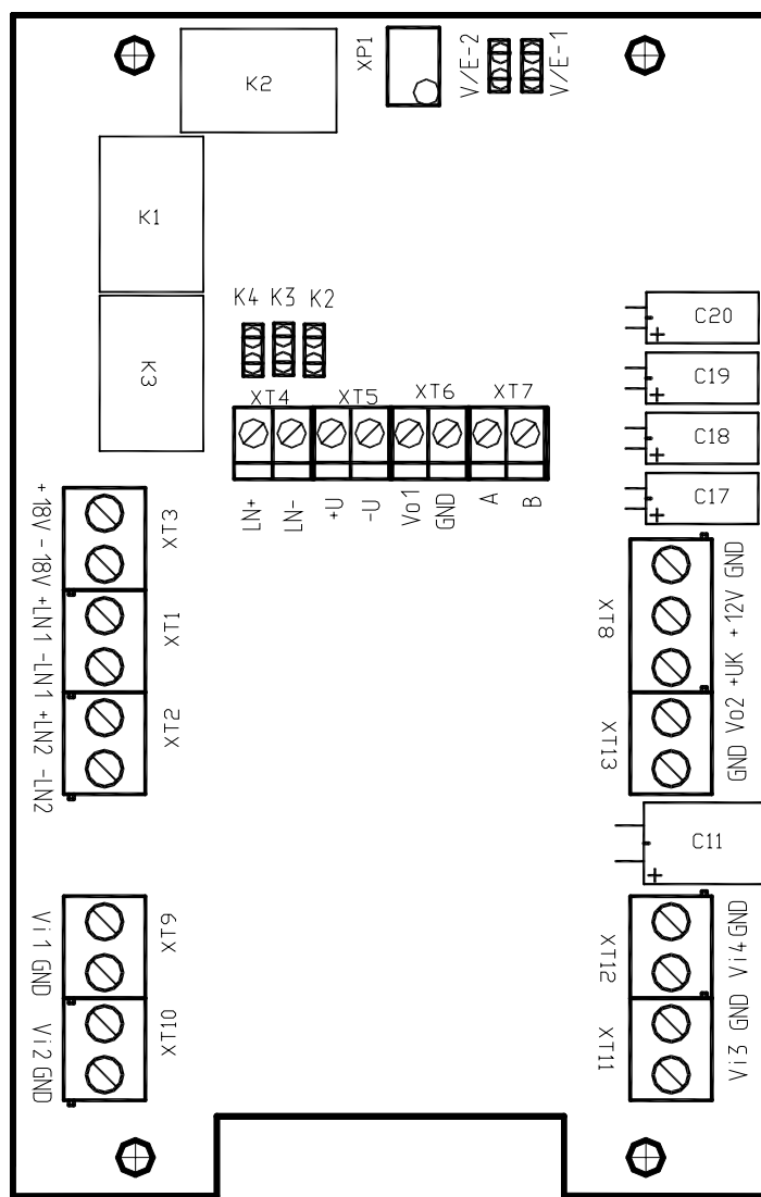
Рис. 15. Внешний вид платы коммутатора.
