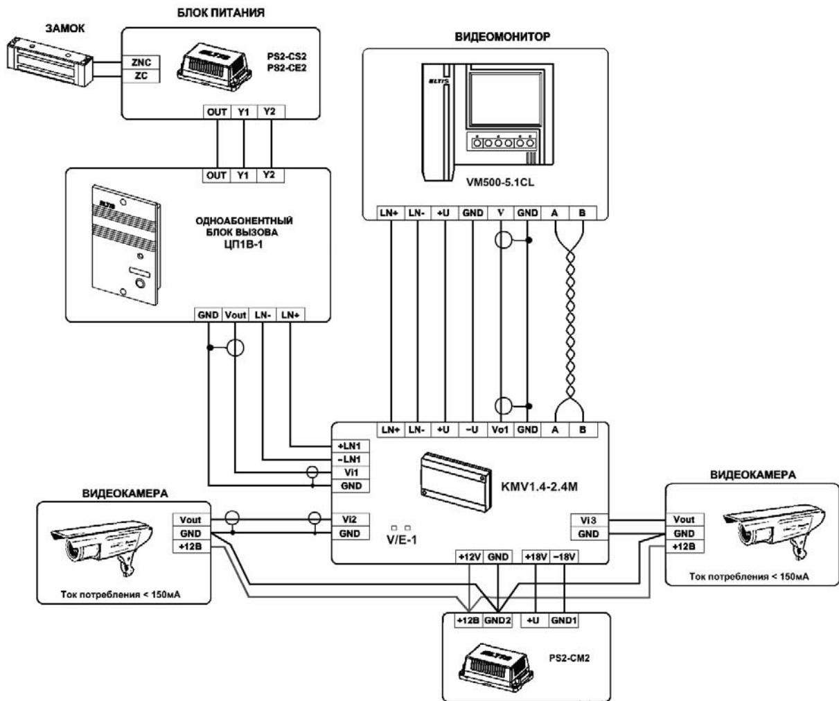
Рис.10 Схема подключения видеомонитора к малоабонентному блоку вызова серии ЦП с 2-мя дополнительными видеосъёмками и коммутатором КМВ1.4-2.4М
