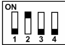
Рис.6 Положение движков переключателя конфигурации при работе видеомонитора без коммутатора типа КМV1.4-2.4(М).
