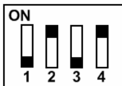
Рис.12 Положение движков переключателя конфигурации при работе с БВ «VIZIT» без коммутатора типа КМV1.4-2.4(М).
