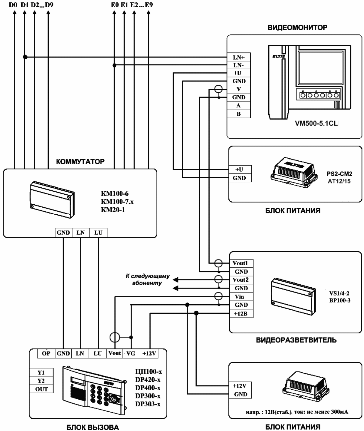
Рис.7 Схема подключения видеомонитора к многоабонентной системе
