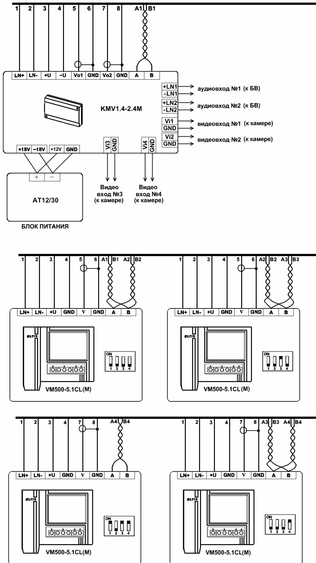
Рис. 13 Пример подключения 4-х видеомониторов к коммутатору KMV1.4-2.4M.
