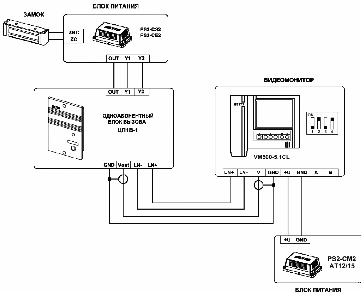
Рис.8 Схема подключения видеомонитора к малоабонентной системе серии ЦП.
