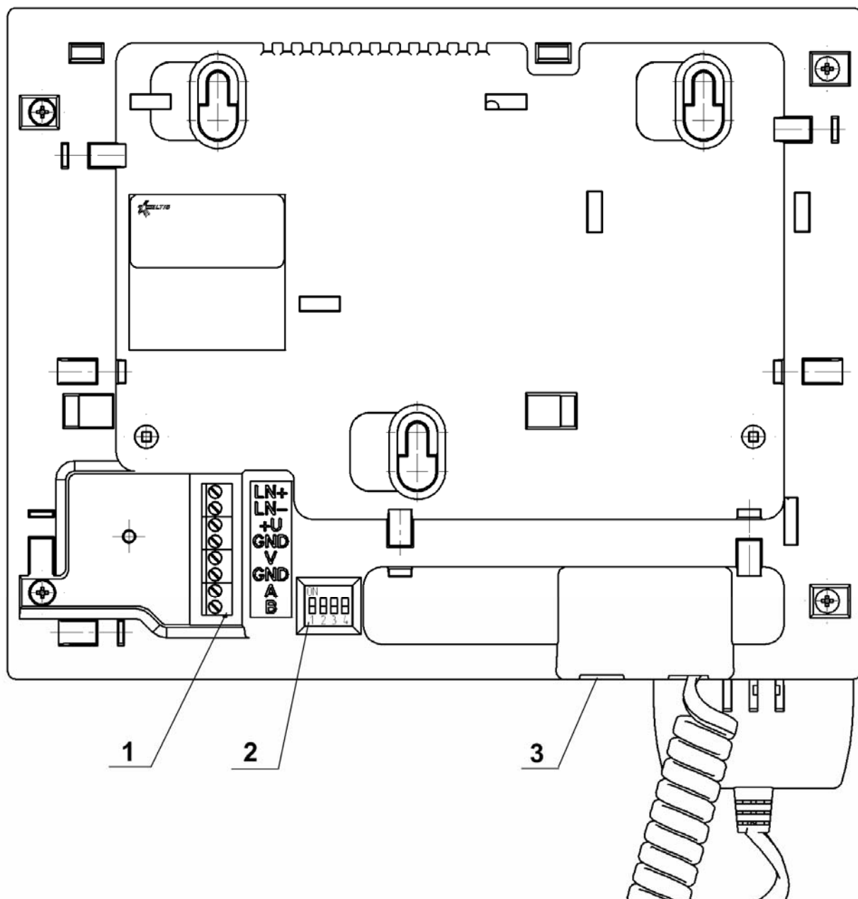
Рис.2: Вид с обратной стороны видеомонитора.
