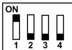
Рис.9 Положение движков переключателя конфигурации при работе с коммутатором типа КМВ1.4-2.4(М).
